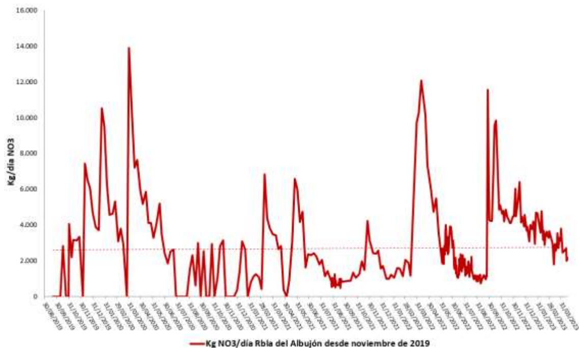
Kg NO 3 /día DESAGUADO POR LA DESEMBOLCADURA DE LA RBLA. DEL ALBUJÓN DESDE NOVIEMBRE 2019
