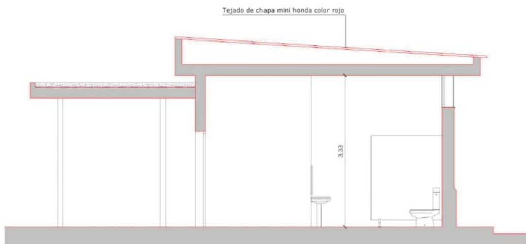
Sección B-B. Estado reformado
